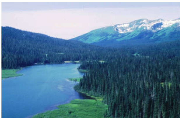
Figure 12. Wet subalpine forest, Kuldo Lake, Skeena.
